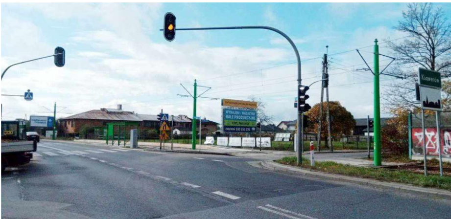
Fotografia przedstawia sygnalizację świetlną na skrzyżowaniu ulicy Łódzkiej/Mały Skręt. Fotografie wykonała redakcja. Informację przygotowała redakcja.
